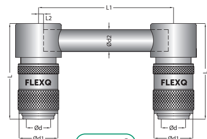
Diverting sockets / Umlenkcupplung
